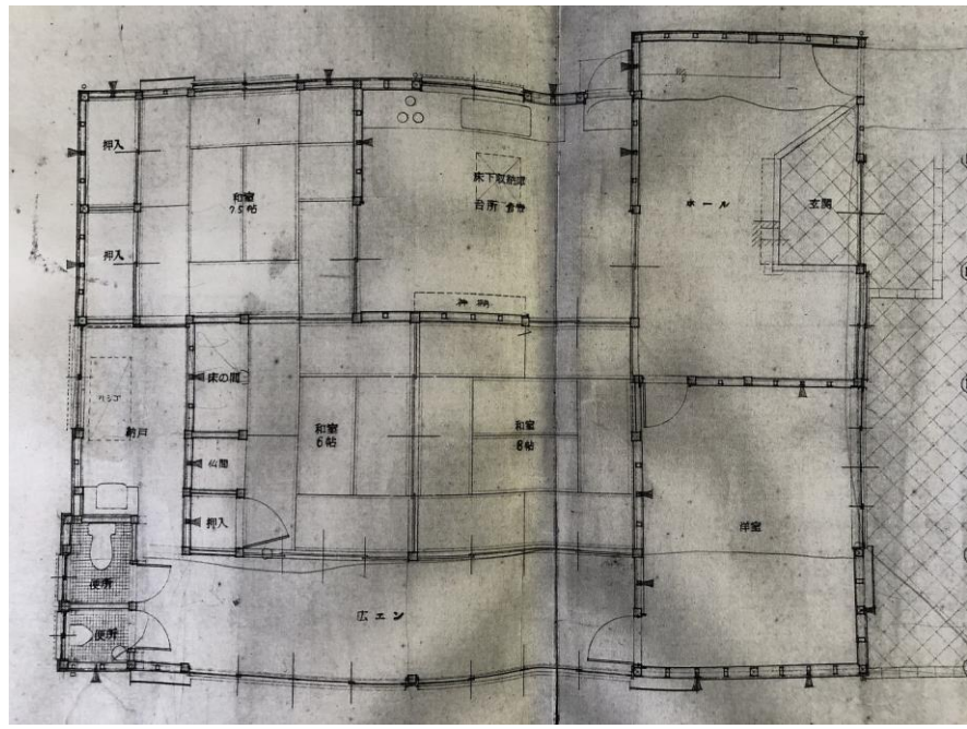
平面図 (間取図)
